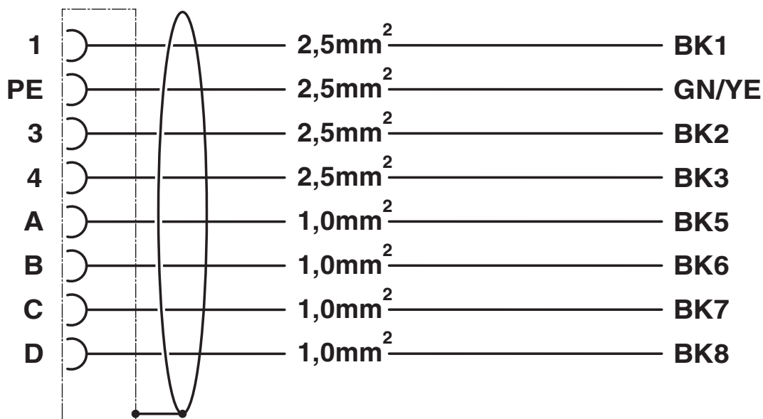
Schemat
