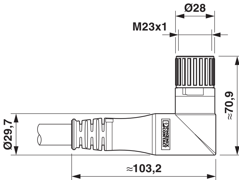
Rysunek wymiarowy
