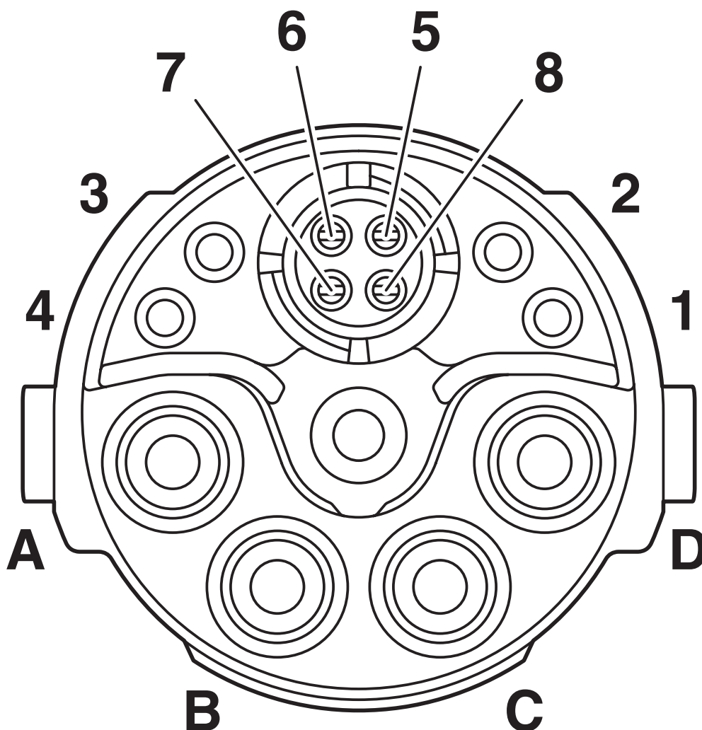
Rysunek schematyczny
