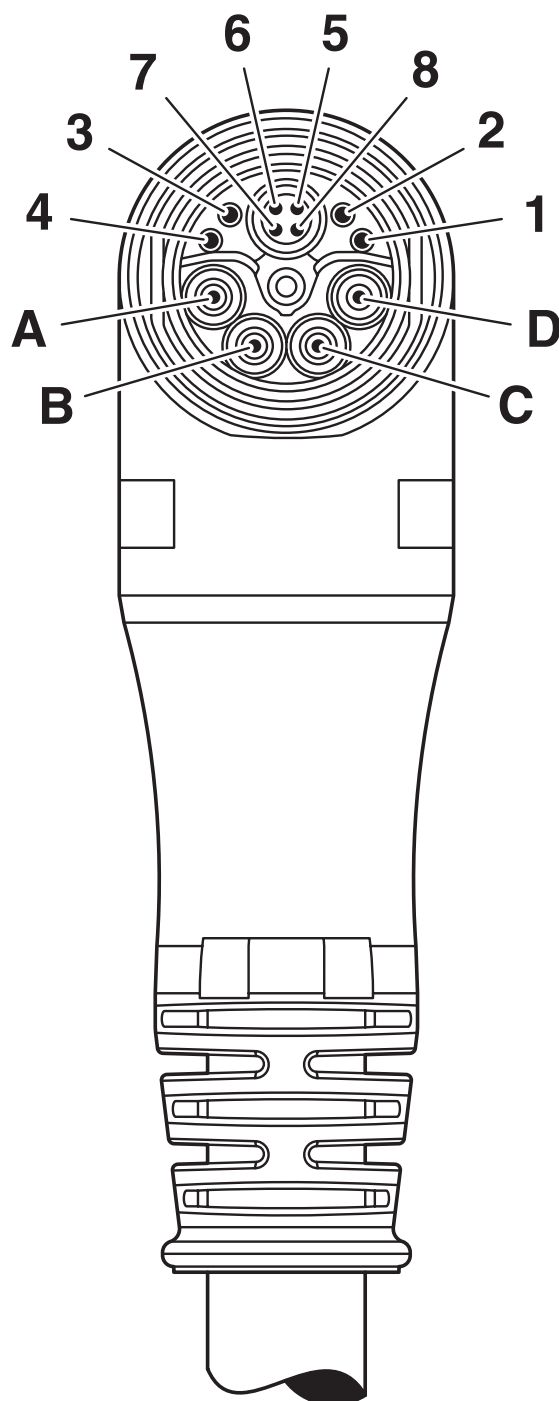
Rysunek schematyczny
