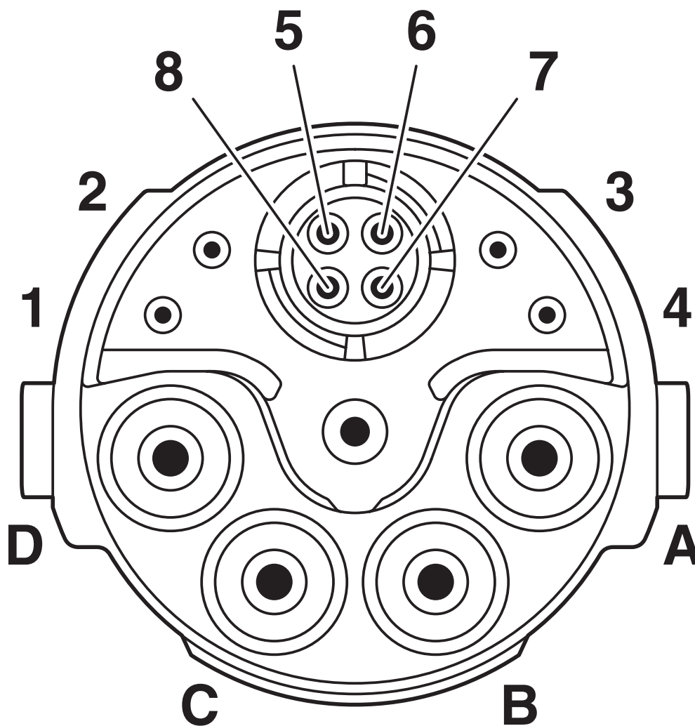
Rysunek schematyczny
