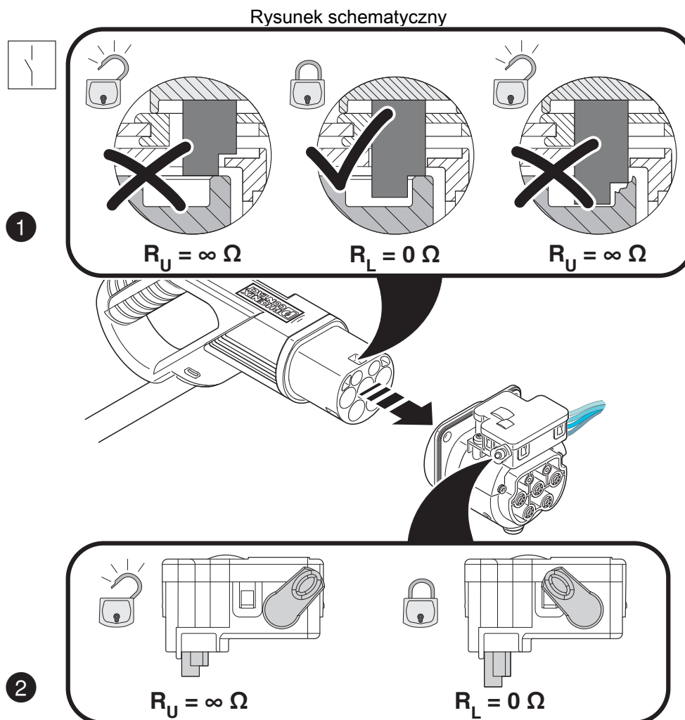
Rysunek schematyczny
