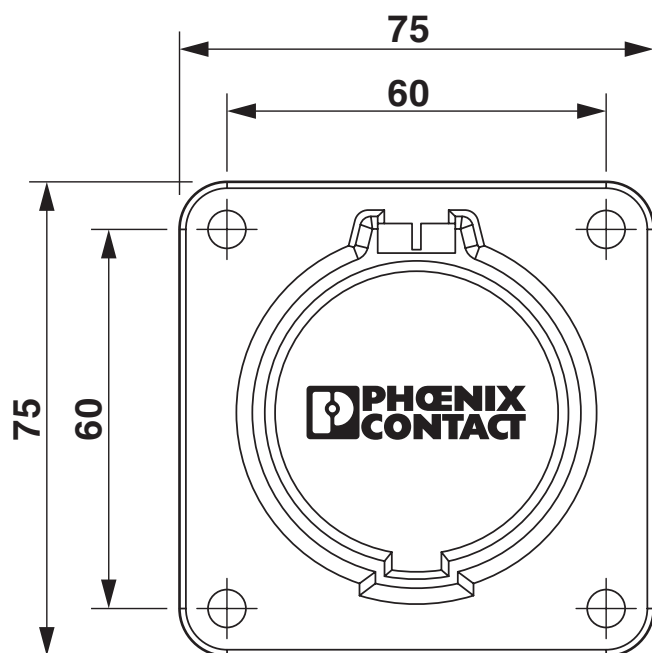
Rysunek wymiarowy
