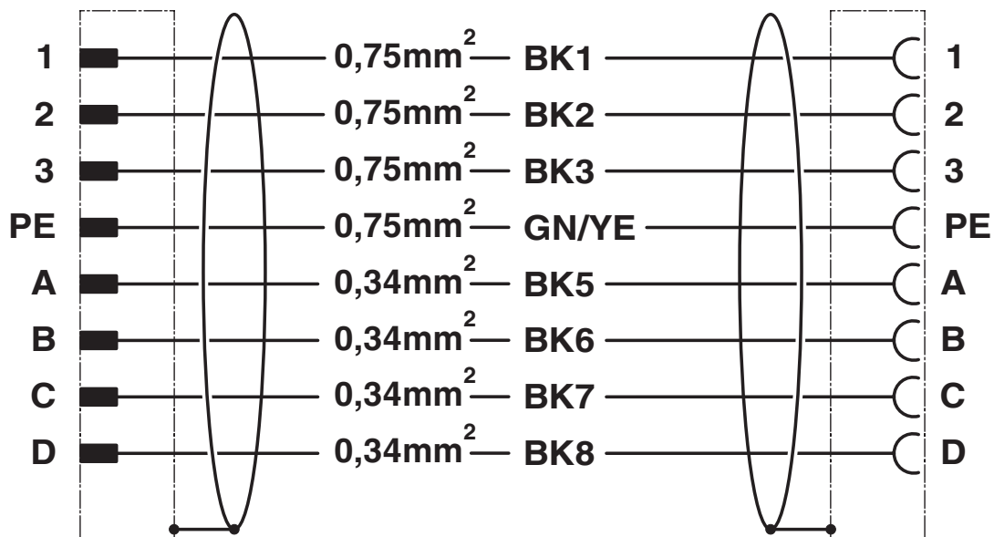
Schemat
