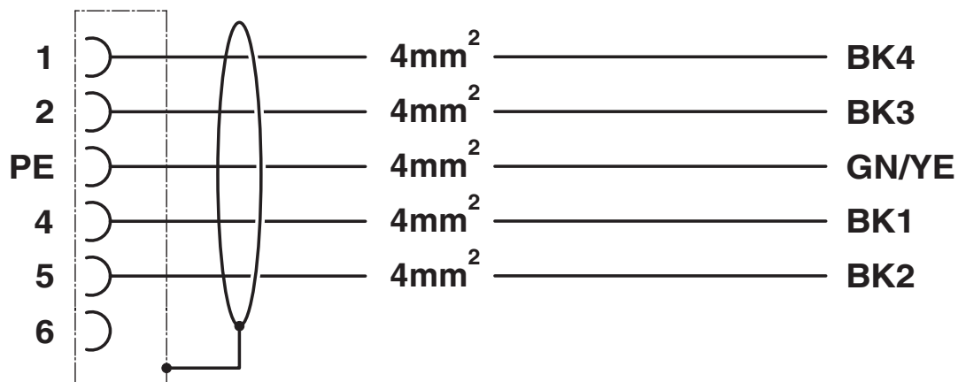
Schemat
