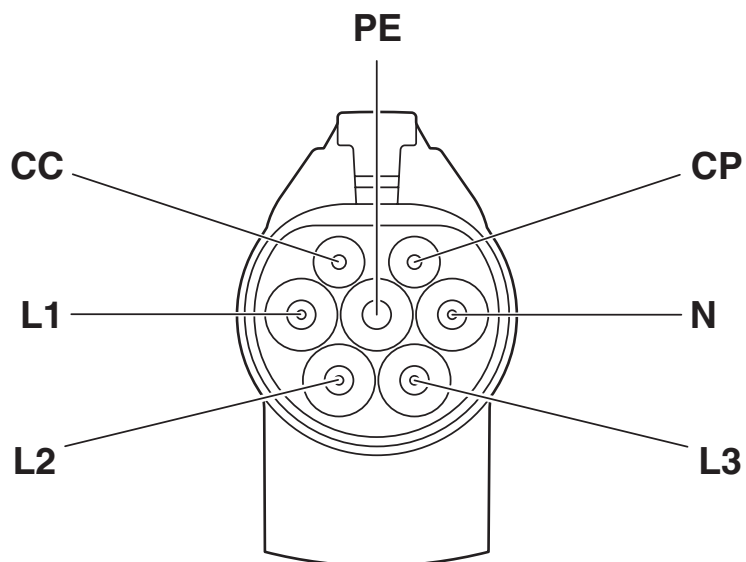
Rysunek schematyczny
