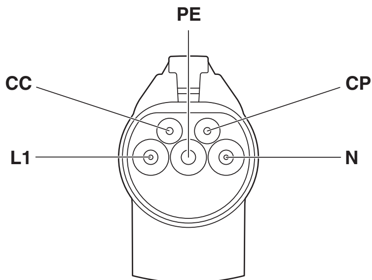
Rysunek schematyczny
