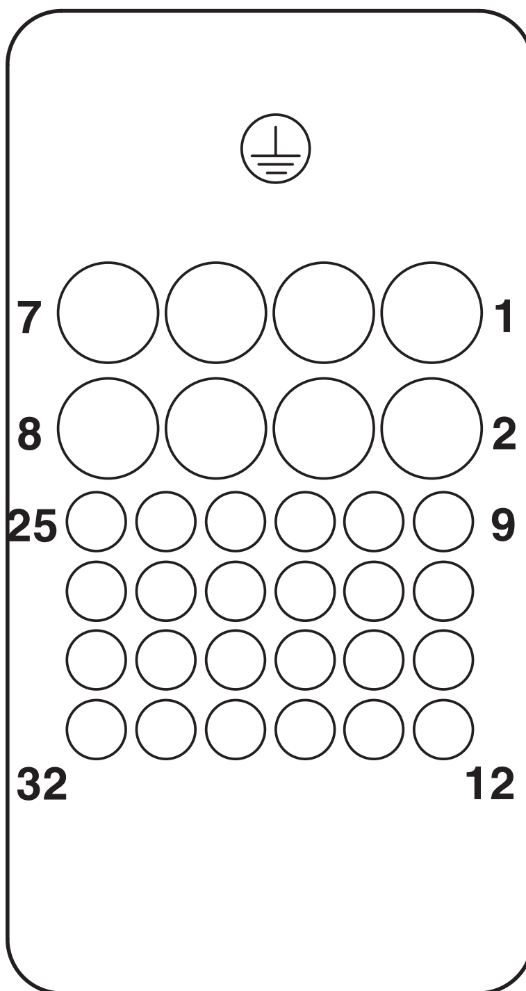
Rysunek schematyczny
