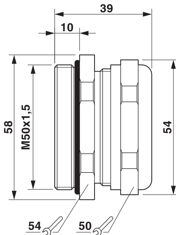
Rysunek wymiarowy
