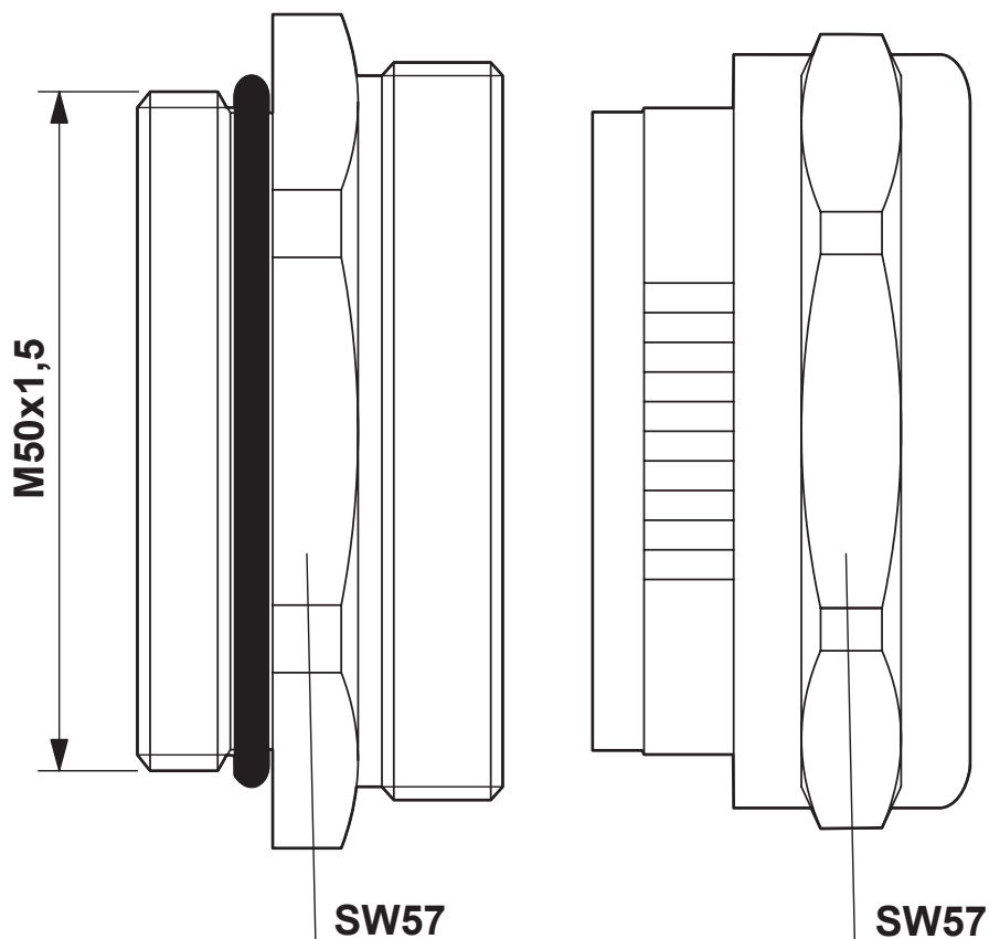
Rysunek wymiarowy
