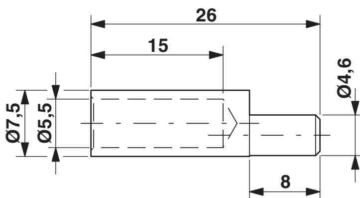
Rysunek wymiarowy
