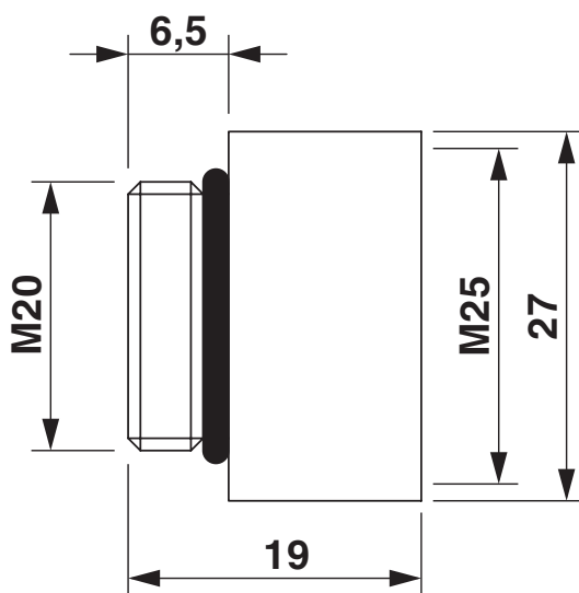
Rysunek wymiarowy
