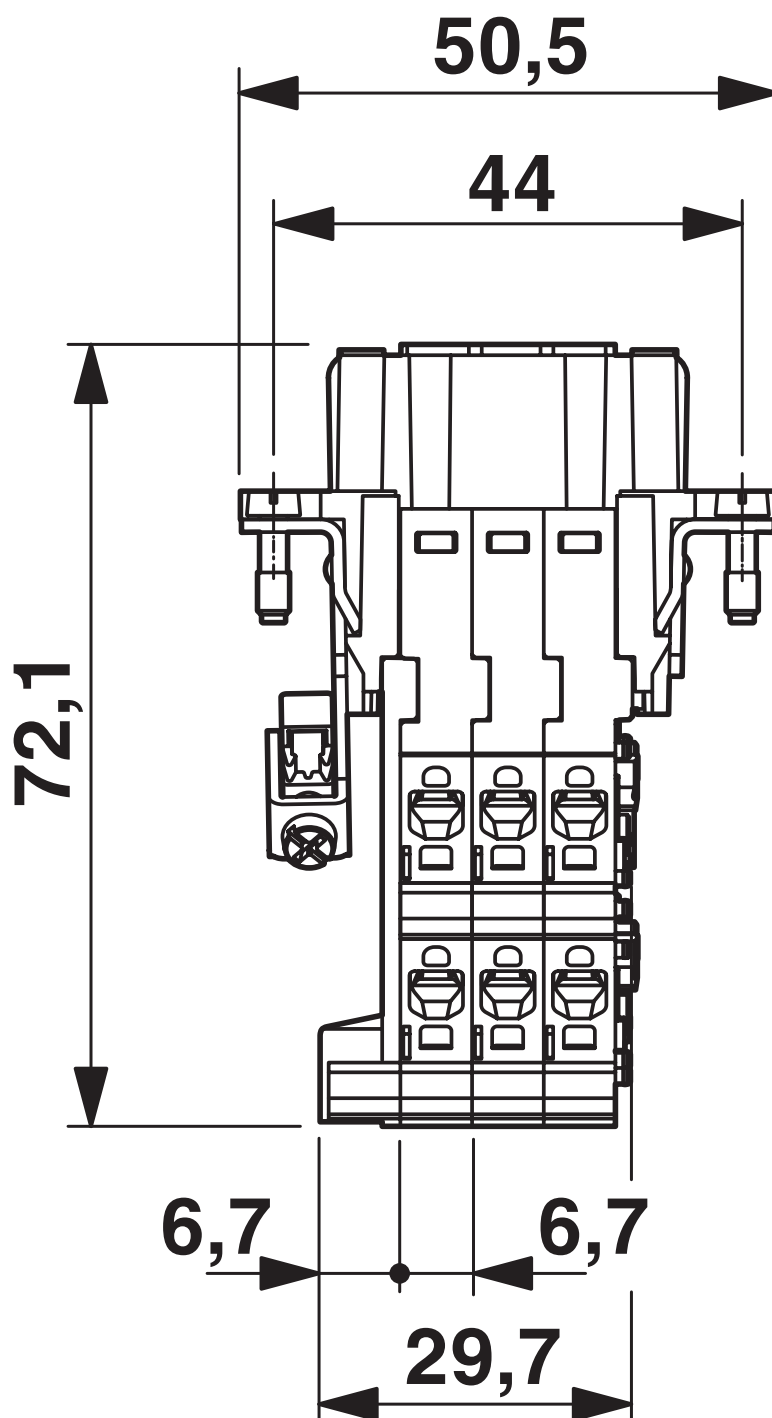
Rysunek wymiarowy
