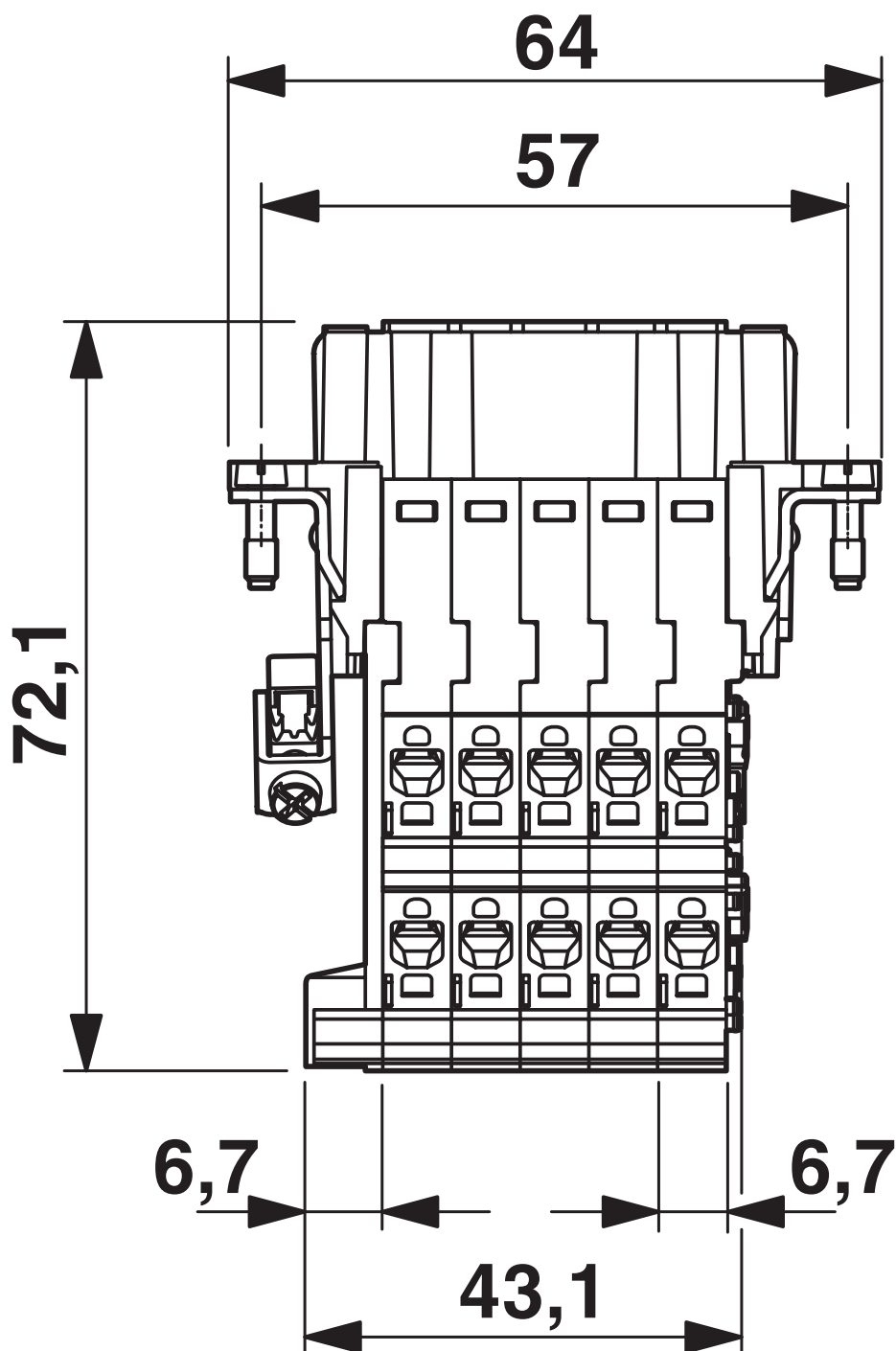
Rysunek wymiarowy
