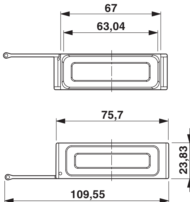
Rysunek wymiarowy
