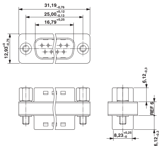
Rysunek wymiarowy
