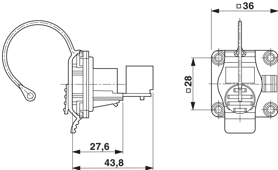
Rysunek wymiarowy
