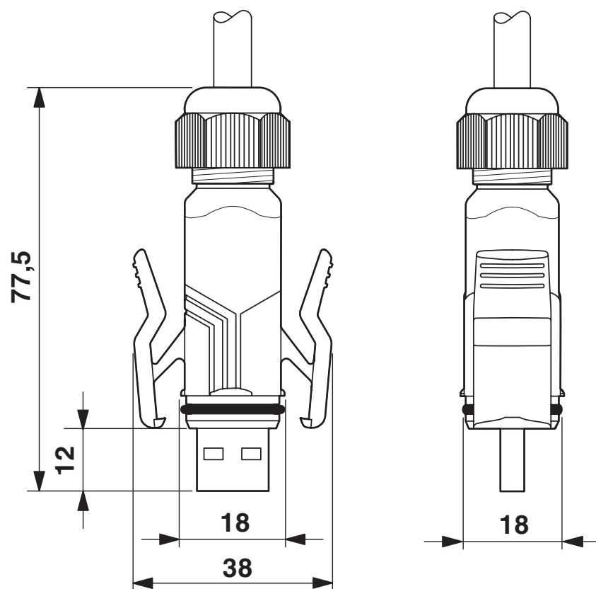
Rysunek wymiarowy
