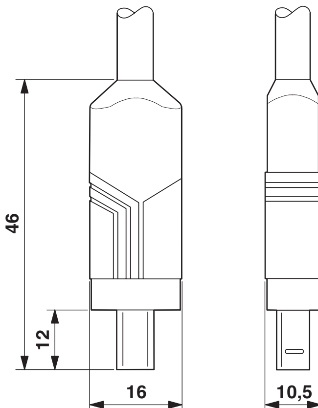
Rysunek wymiarowy
