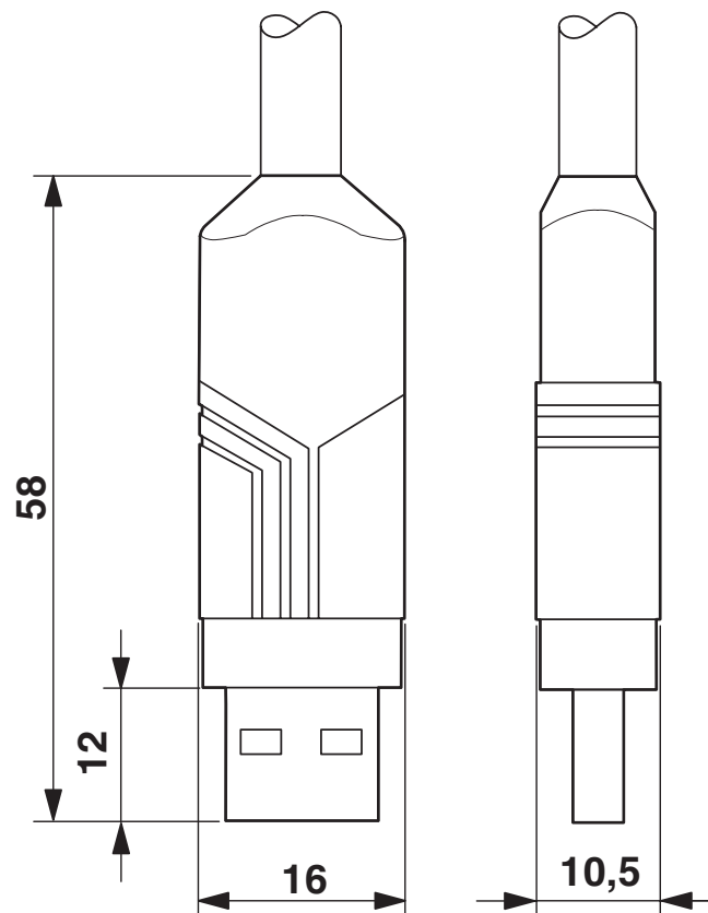
Rysunek wymiarowy
