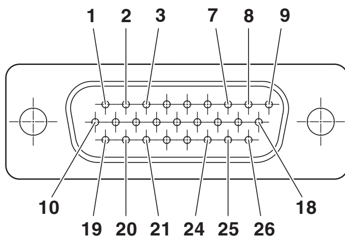
Rysunek schematyczny
