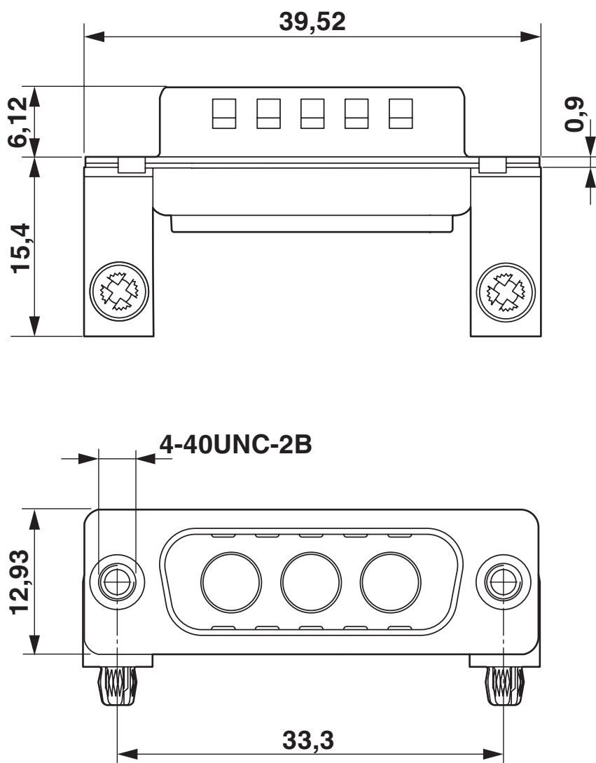
Rysunek wymiarowy
