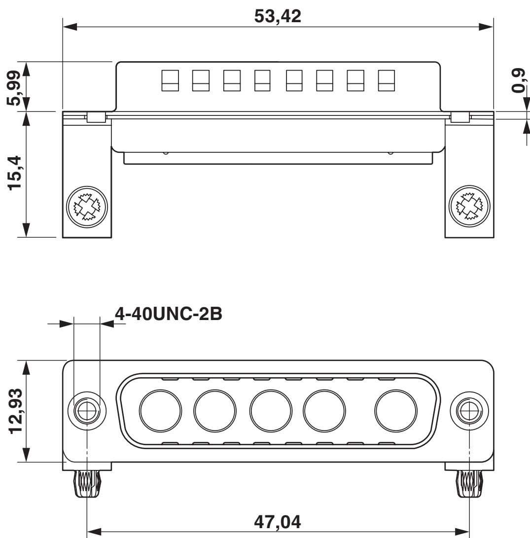
Rysunek wymiarowy
