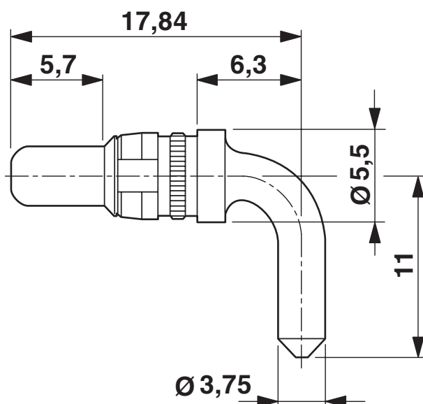
Rysunek wymiarowy
