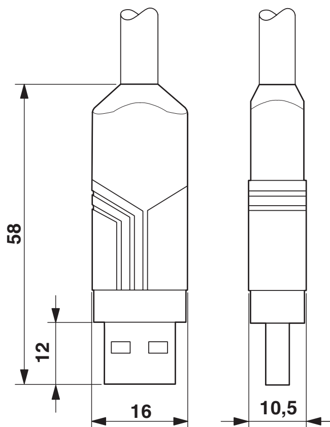
Rysunek wymiarowy
