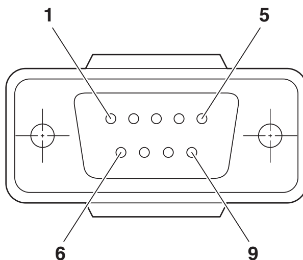
Rysunek schematyczny
