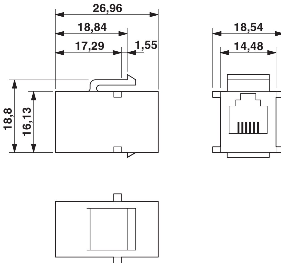
Rysunek wymiarowy
