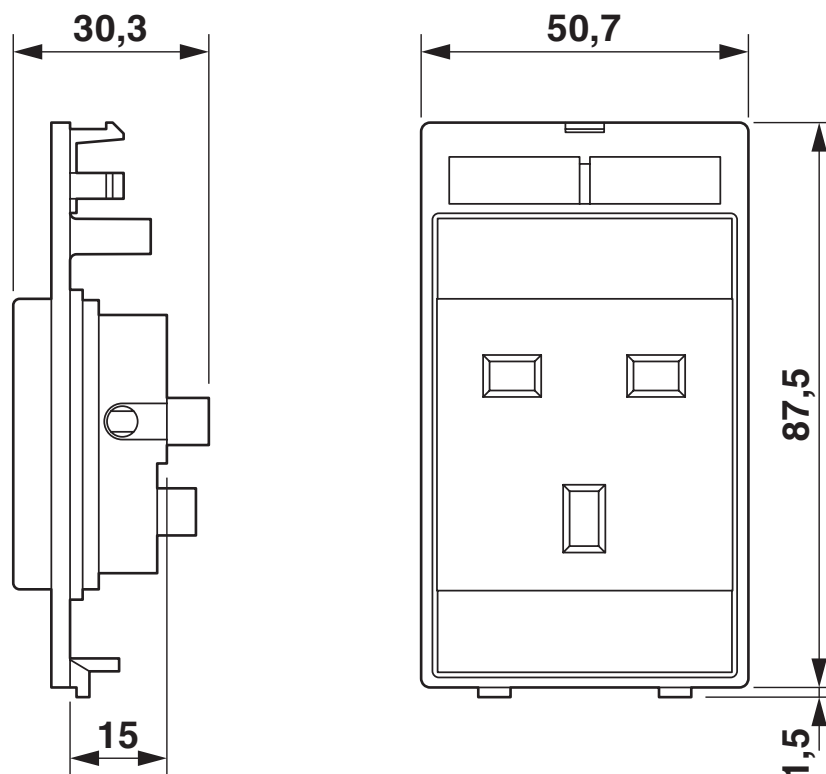
Rysunek wymiarowy
