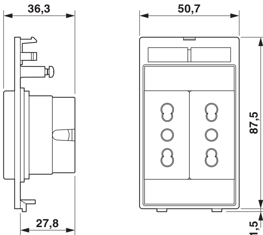
Rysunek wymiarowy
