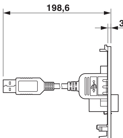
Rysunek wymiarowy
