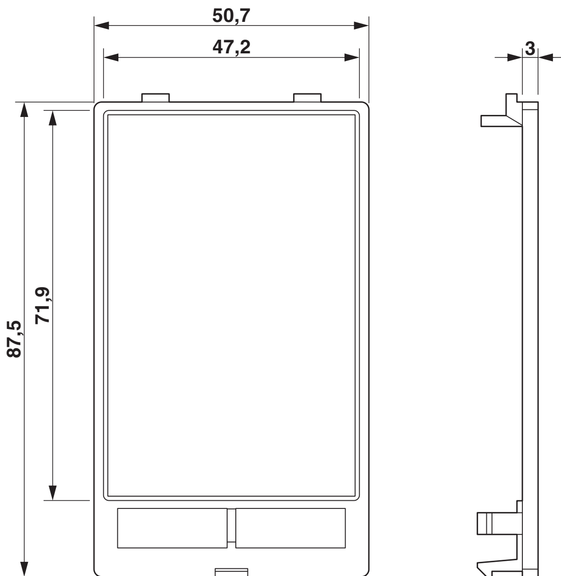
Rysunek wymiarowy
