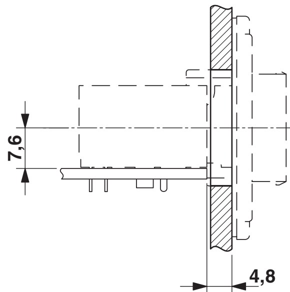
Rysunek wymiarowy
