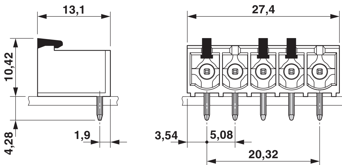
Wkładka styków MSTB
