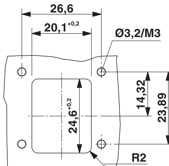
Rysunek wymiarowy
