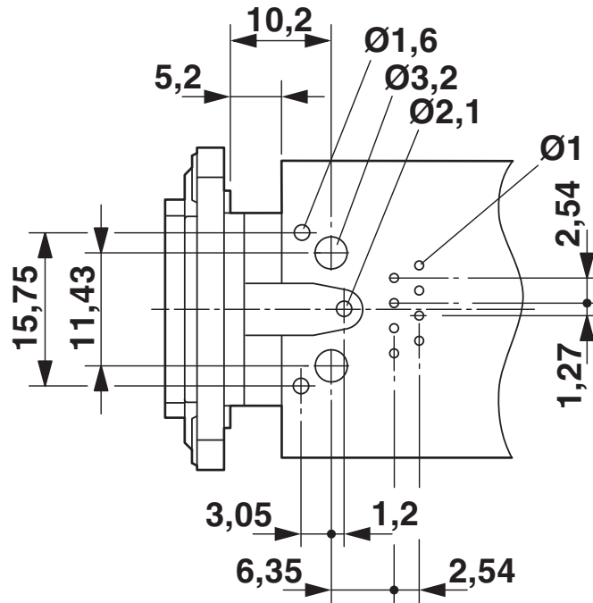
Otworowanie/geometria płytek lutowniczych
