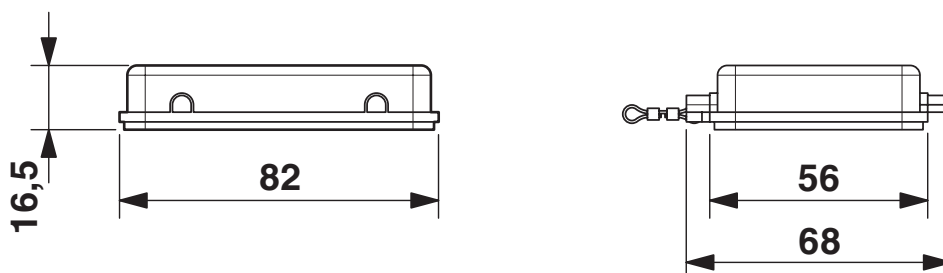
Rysunek wymiarowy
