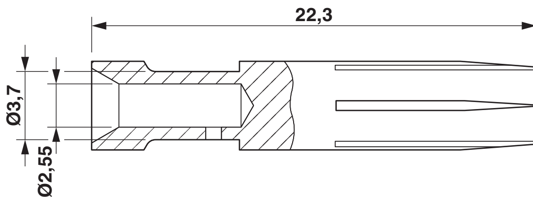
Rysunek wymiarowy
