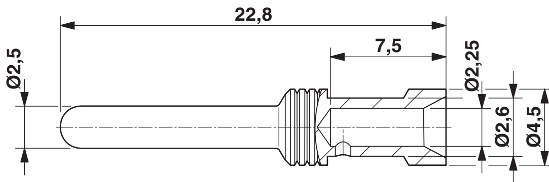
Rysunek wymiarowy
