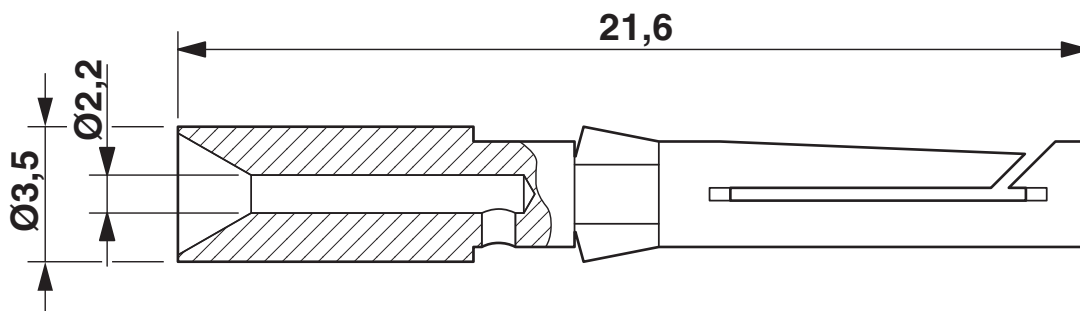
Rysunek wymiarowy
