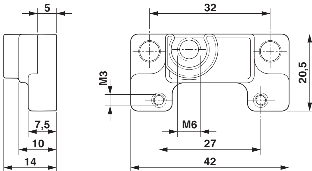
Rysunek wymiarowy
