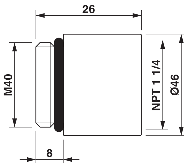
Rysunek wymiarowy
