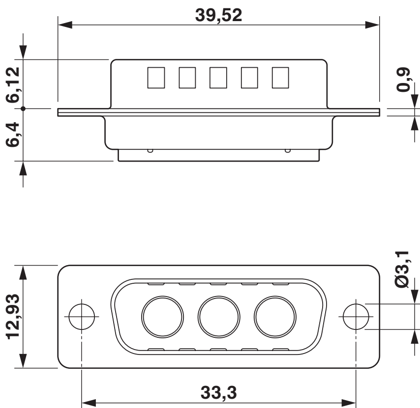
Rysunek wymiarowy
