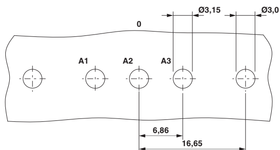
Otworowanie/geometria płytek lutowniczych
