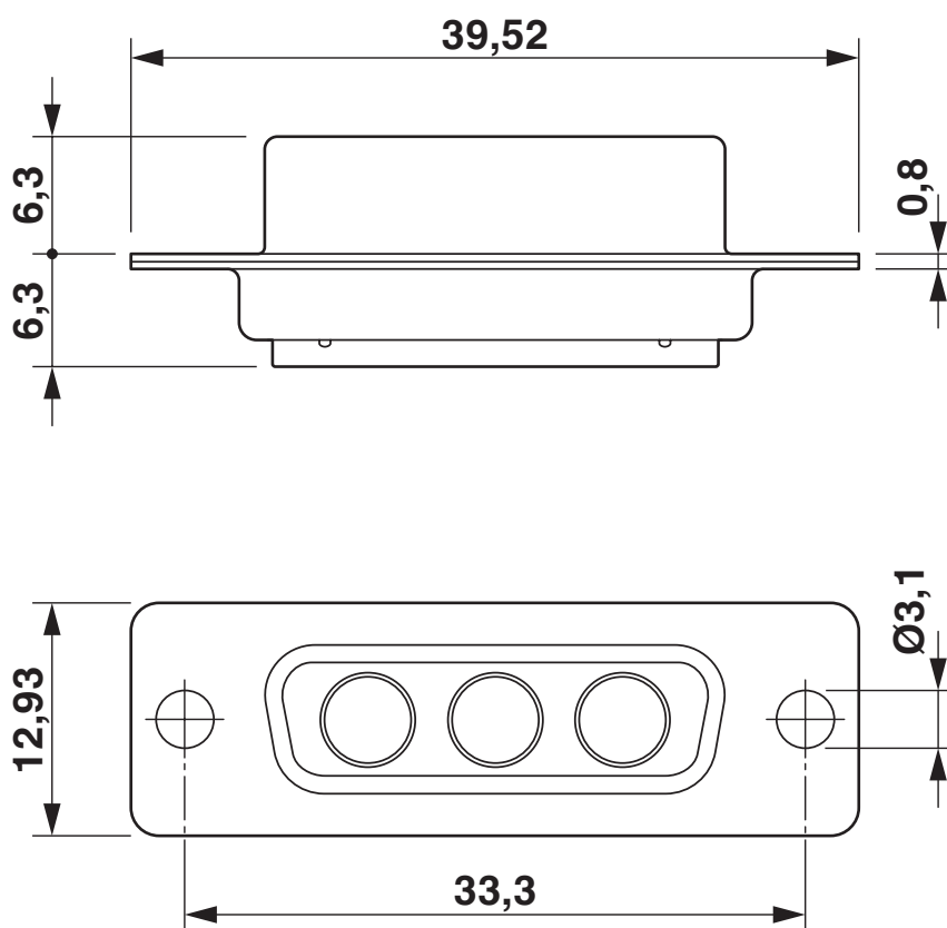
Rysunek wymiarowy
