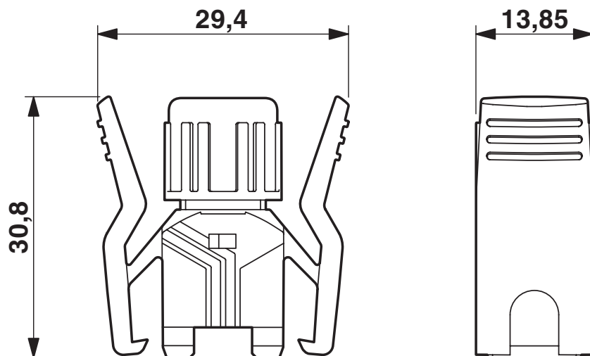
Rysunek wymiarowy
