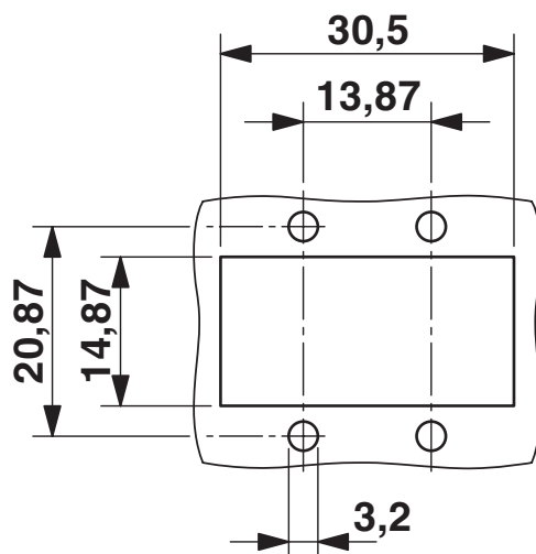
Rysunek wymiarowy
