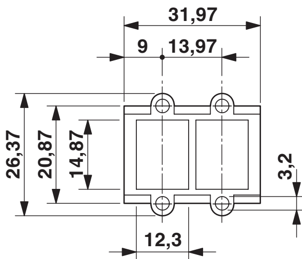
Rysunek wymiarowy
