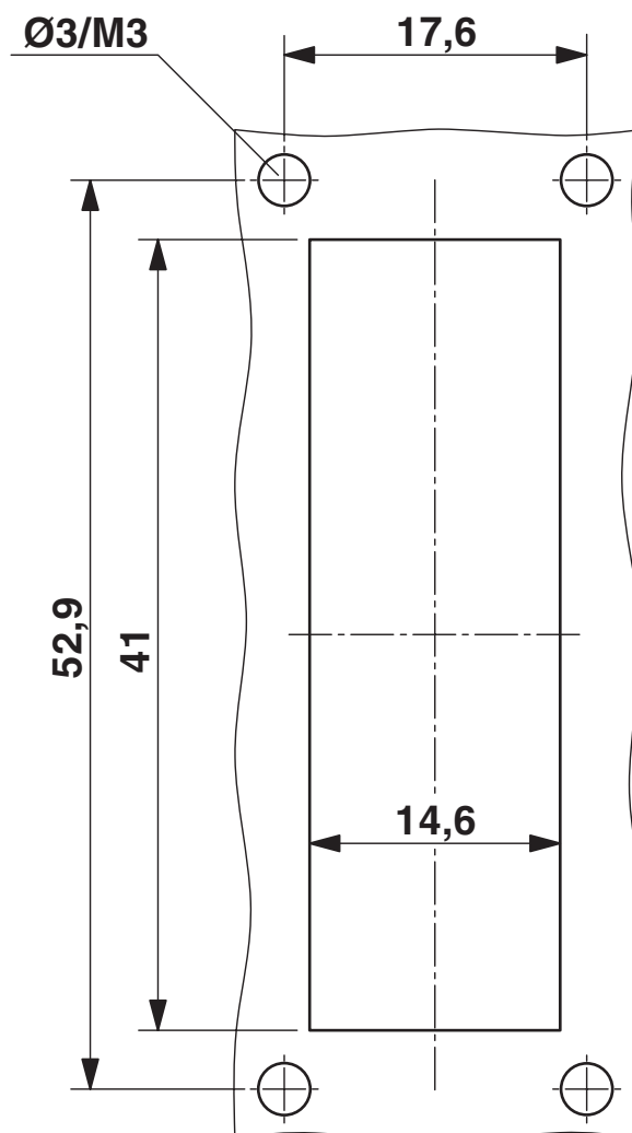
Rysunek wymiarowy
