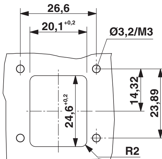
Rysunek wymiarowy
