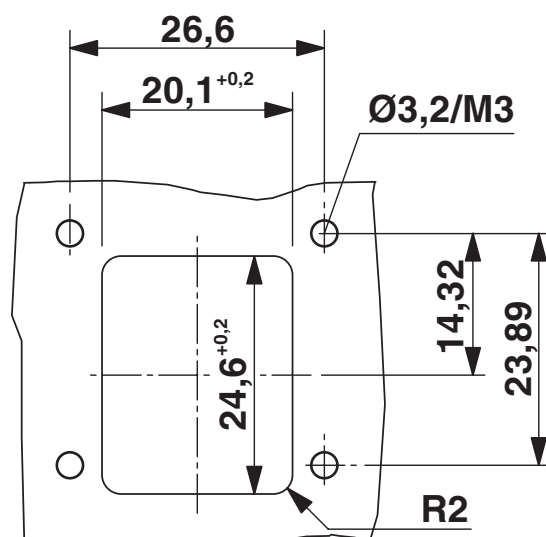
Rysunek wymiarowy
