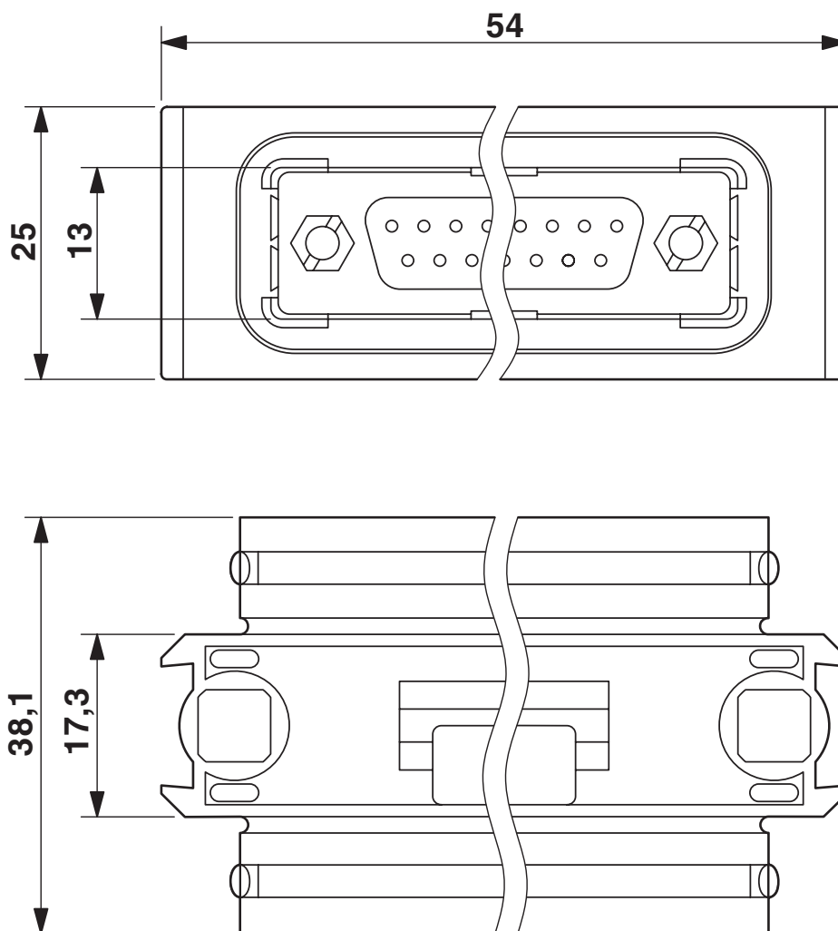
Rysunek wymiarowy
